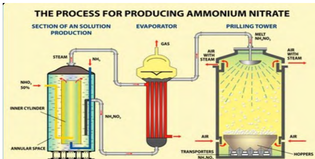
Figure - Principe de production de grains d'ammonitrate par prilling (source : Shutterstock)
