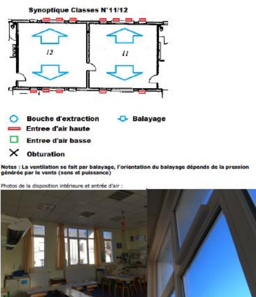
Figure 25: Illustration du système d'aération
