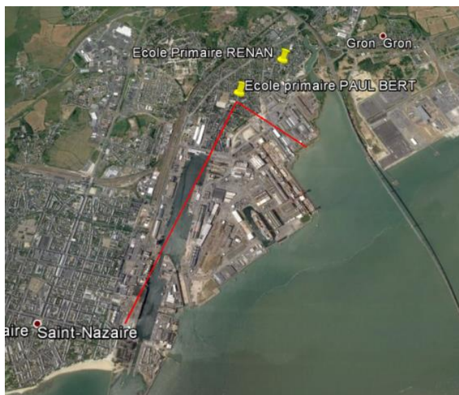
Figure 11: Direction des vents durant les élévations
