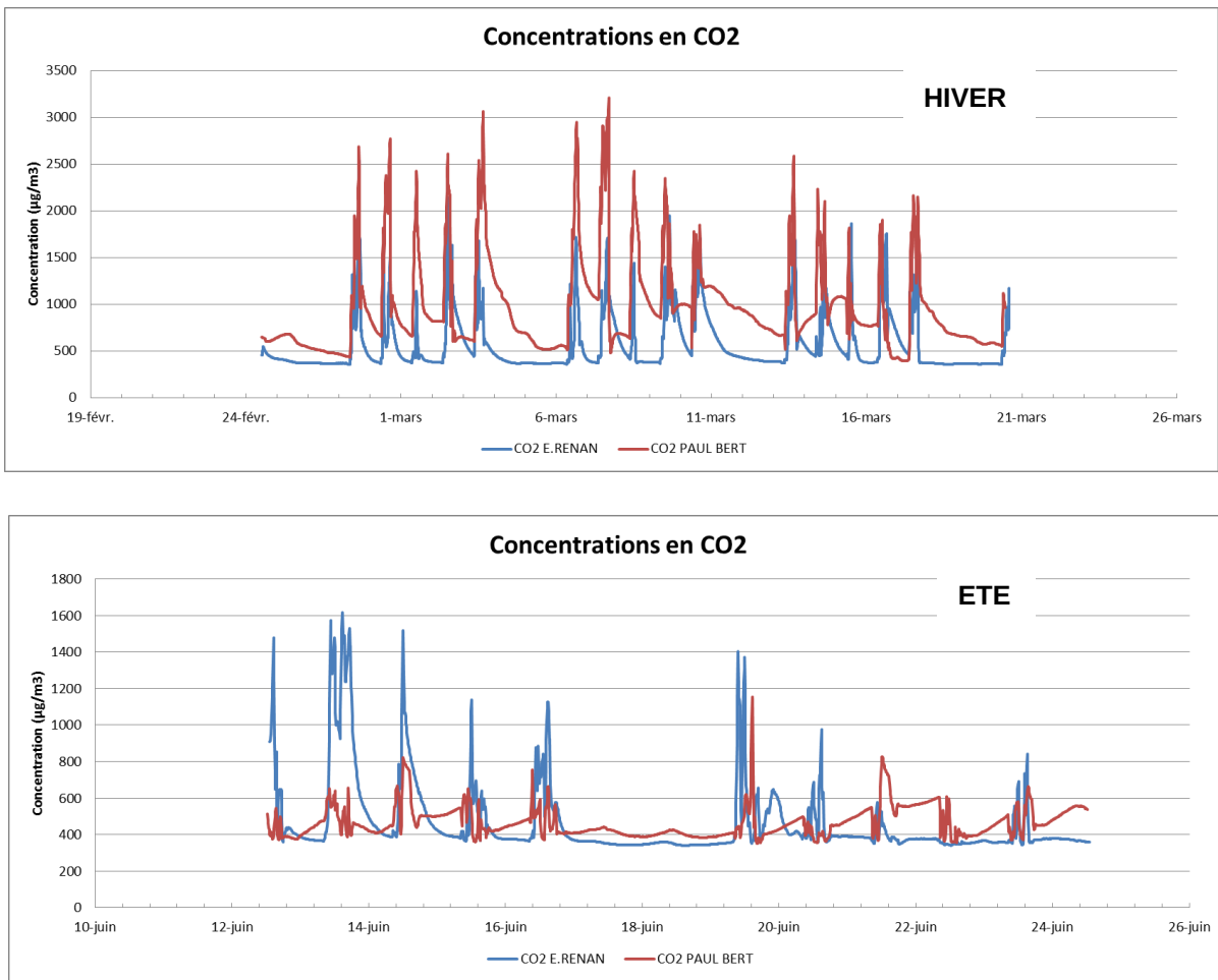
Figure 24: Concentrations en CO 2 dans les salles de classe - campagne hiver et été
