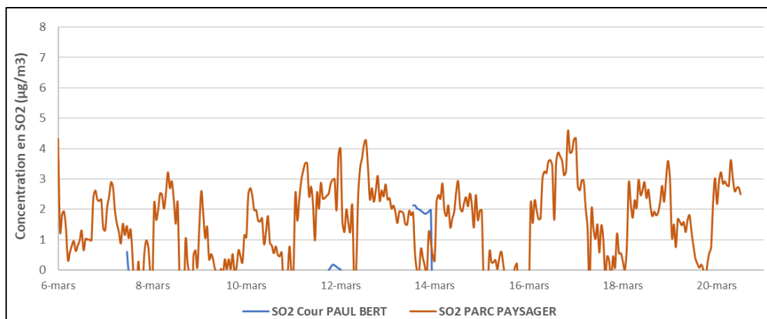
Figure 32: Concentrations en \text{SO}_2 en air extérieur à proximité des écoles instrumentées
