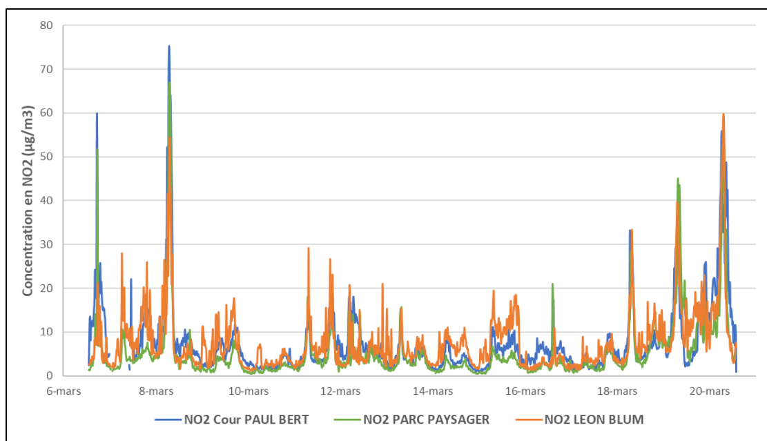
Figure 33: Concentrations en \text{NO}_2 en air extérieur à proximité des écoles instrumentées
