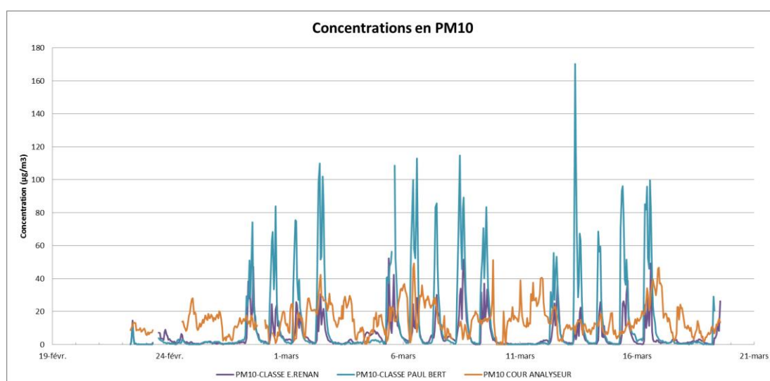
Figure 18: Concentrations horaires en \text{PM}_{10} dans les salles de classe - campagne hiver
