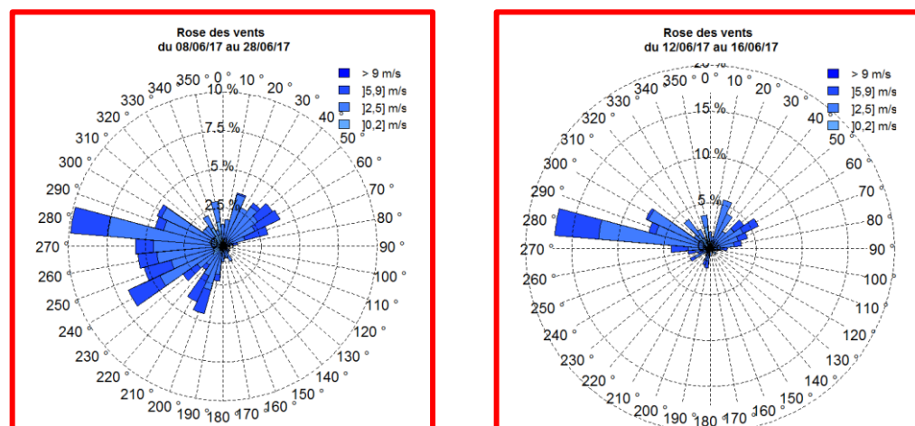
Figure 9: Roses des vents été
